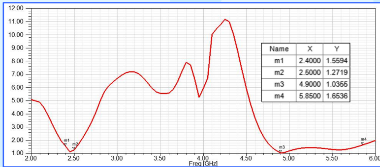
VSWR
