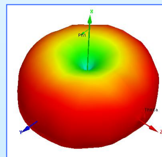
5.55GHz
