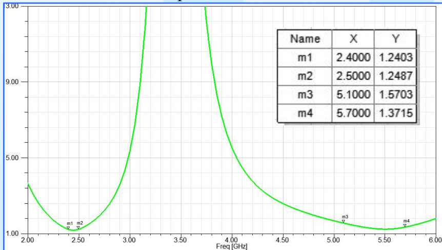
VSWR
