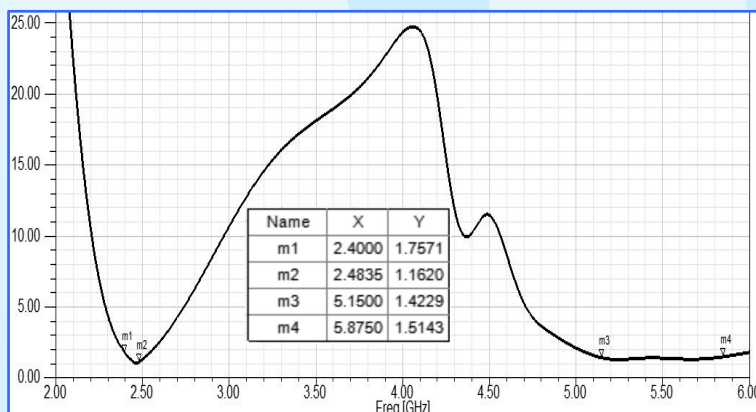
VSWR
