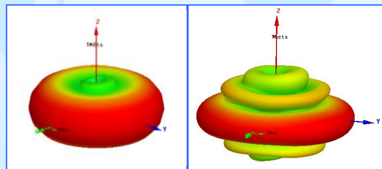
5.55GHz
