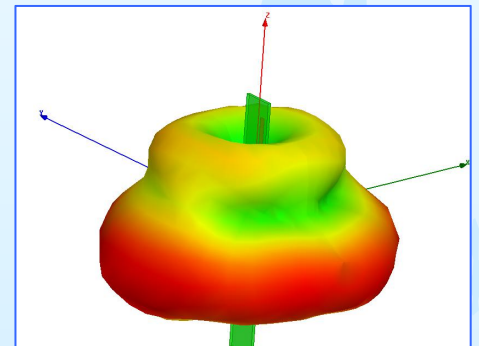
6550MHz
