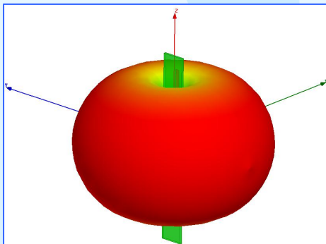
2440MHz
