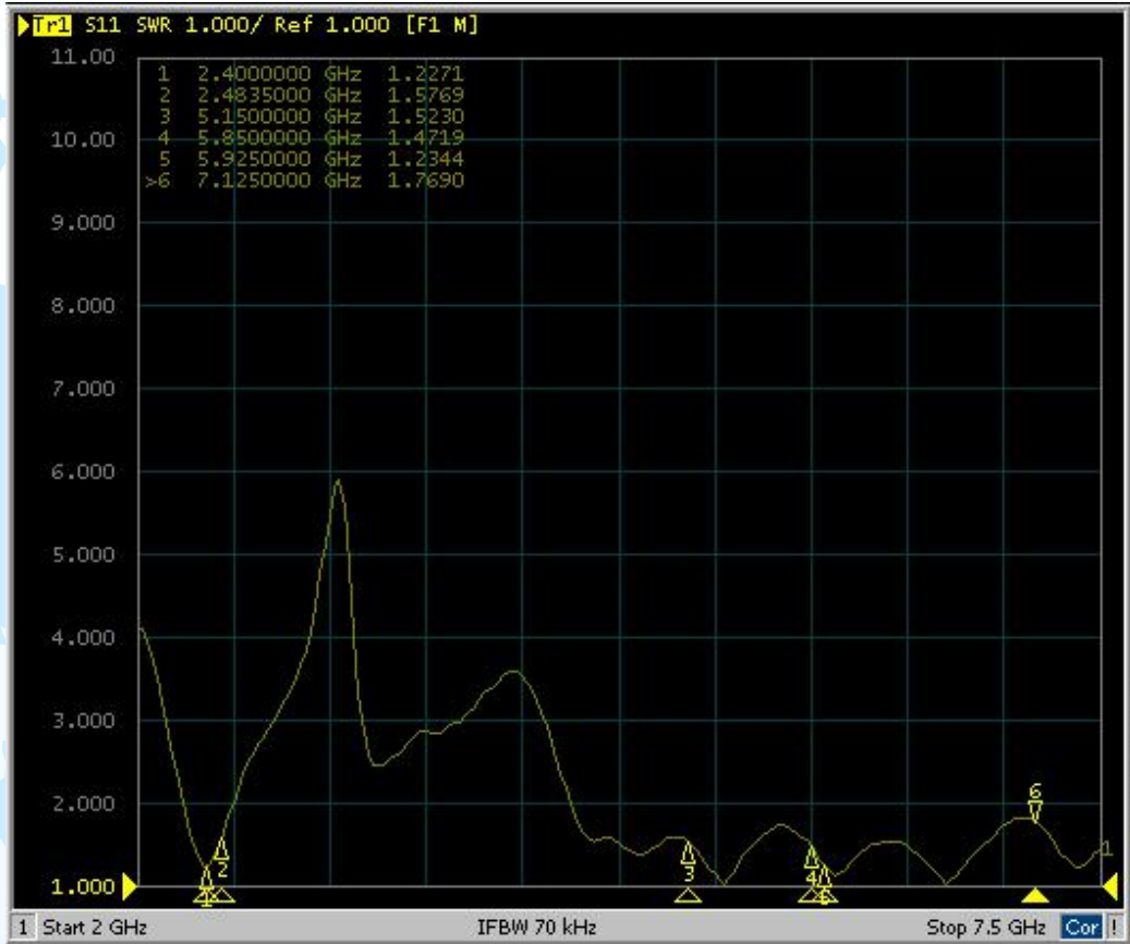
VSWR
