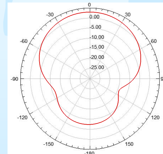
E-面@2492MHz
