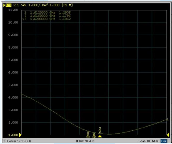
VSWS:L频段
