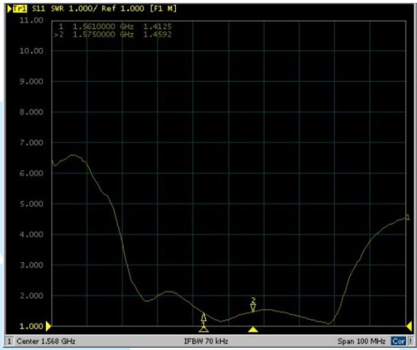
VSWR:B1/L1频段
