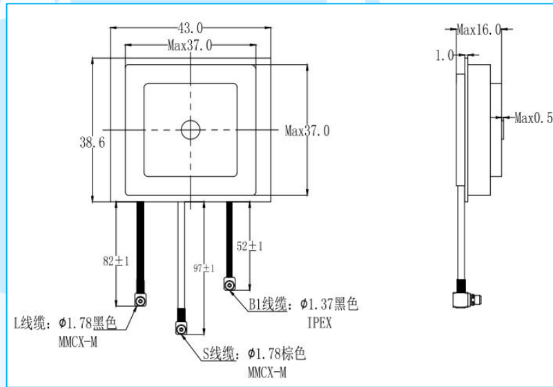
外形图 (单位: mm)
