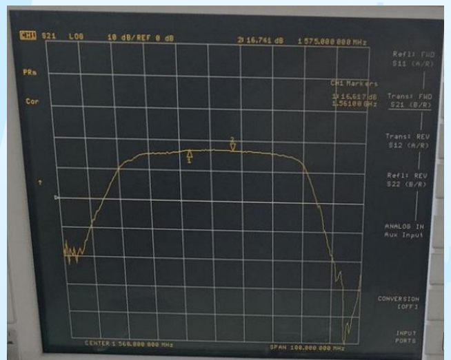
B1/L1有源增益 (加电3.3V)
