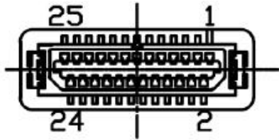
广濂 DF9_25S_1V, 底板需使用 DF9_25P_1V
