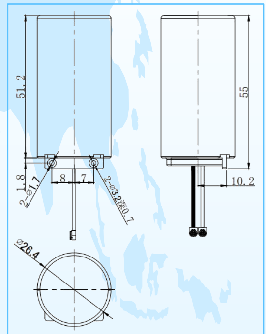
外形图: (单位: mm)
